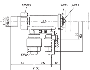
Распределительный клапан с наружной резьбой
