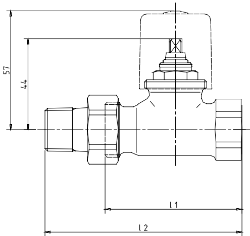
Рис. 2. Прямой.
