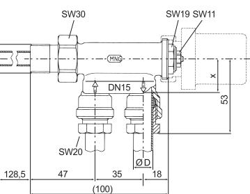
Распределительный клапан с инжекторной трубкой и внутренней резьбой
