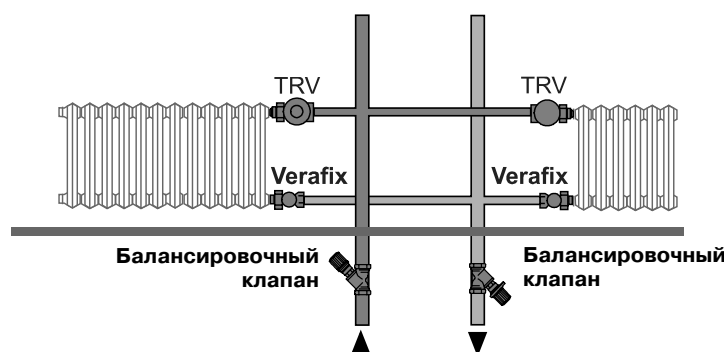
Рис. 3. Пример установки.
