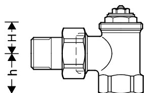
Рис. 1. Угловой.
