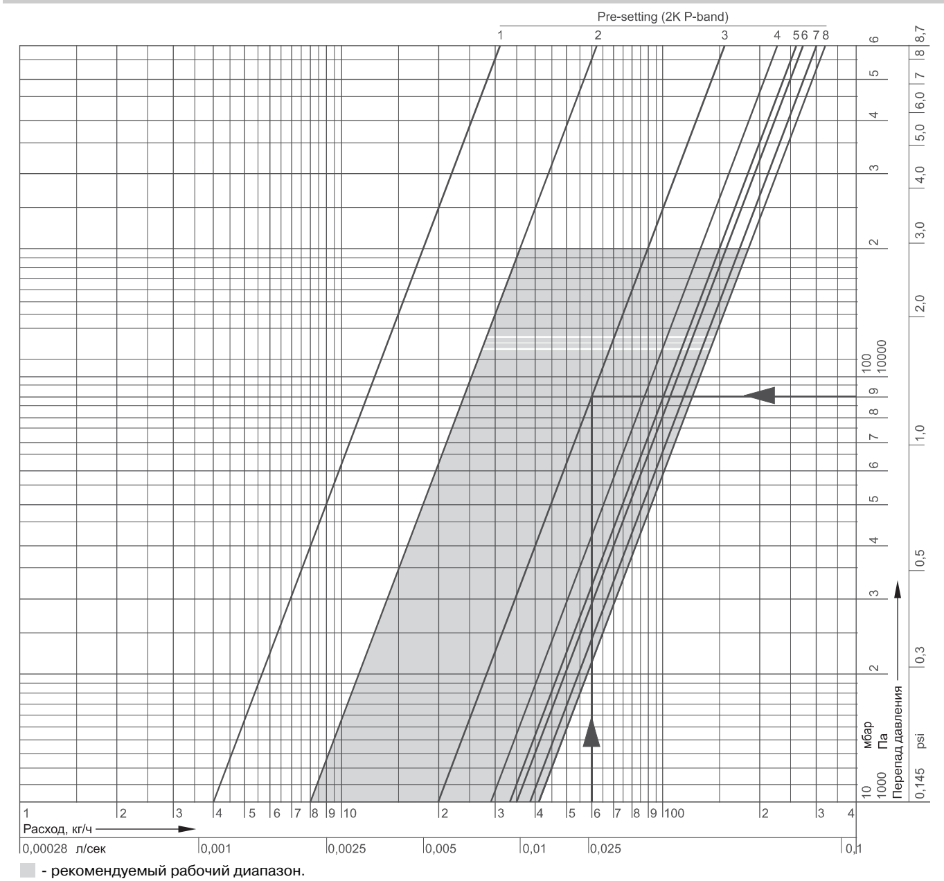
ДИАГРАММА РАСХОДА
