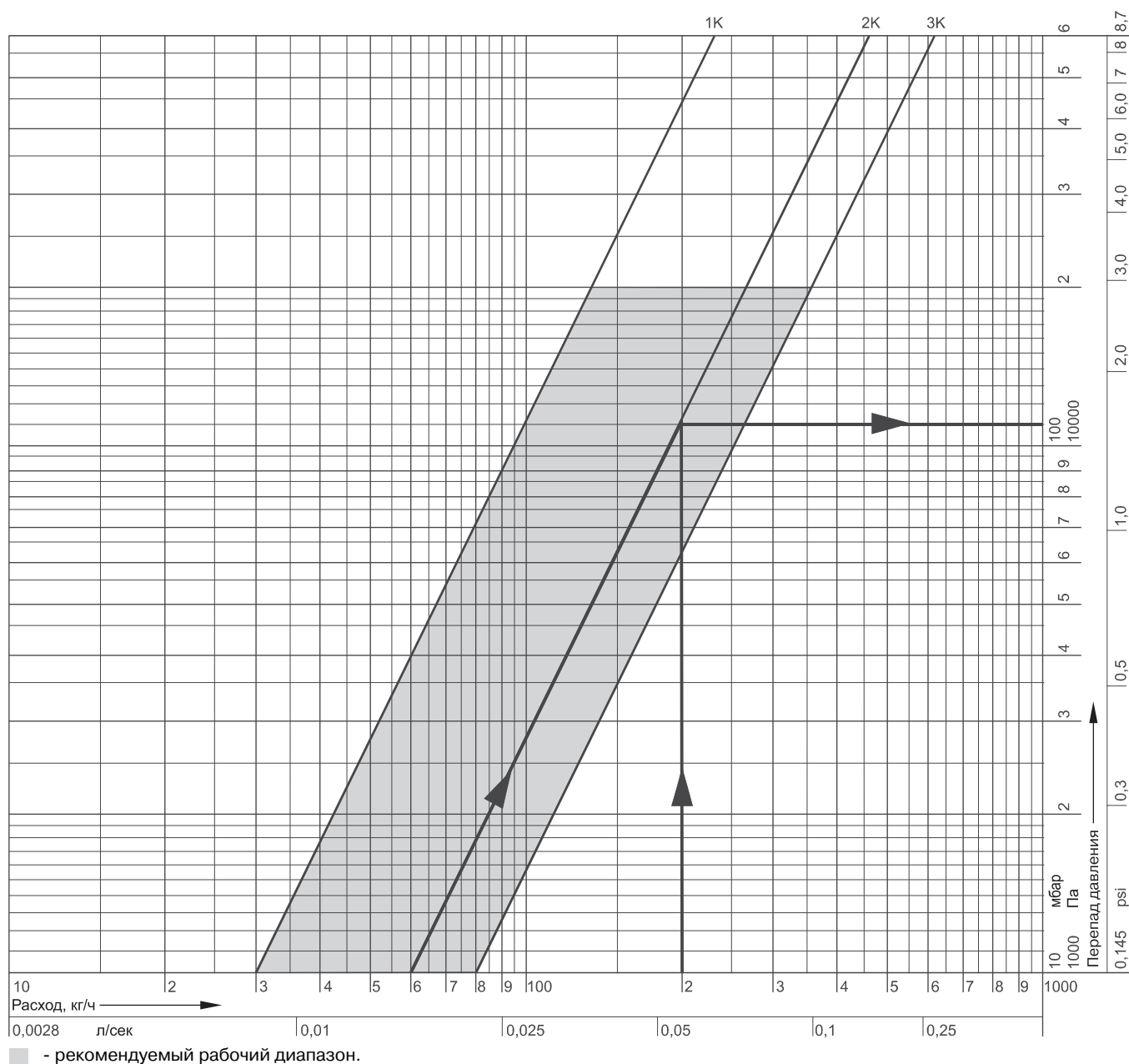
ДИАГРАММА РАСХОДА
