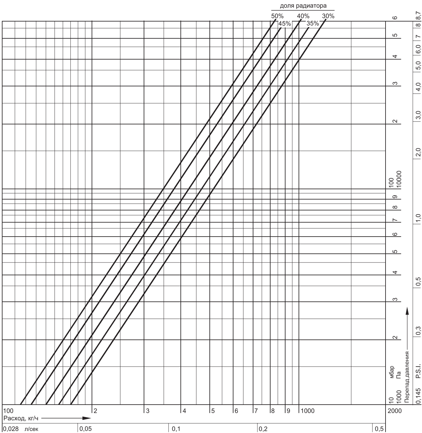
ДИАГРАММА РАСХОДА VERAFIG-VK В 1-НО ТРУБНОЙ СИСТЕМЕ, ПРЯМОЙ.
