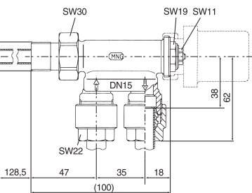
Распределительный клапан с инжекторной трубкой и наружной резьбой
