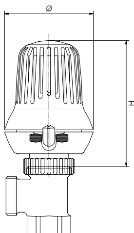
Рис. 1. Tera-3 с встроенным датчиком
