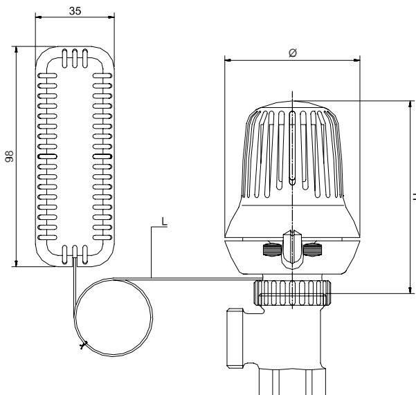
Рис. 2. Tera-3 с дистанционным датчиком
