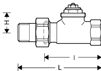
Рис. 2. Прямой.
