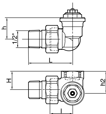
Рис. 4. Угловой торцевой.
