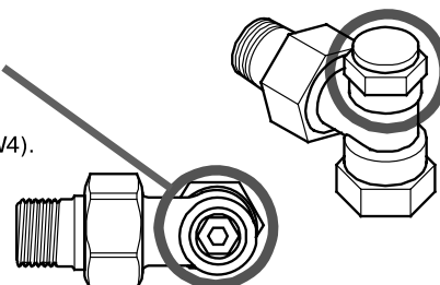
Рис. 5. Идентификация Verafix-E.
