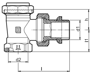
Рис. 1. Угловой с внутренним резьбовым соединением на входе. Рис. 2. Прямой с внутренним резьбовым соединением на входе.
