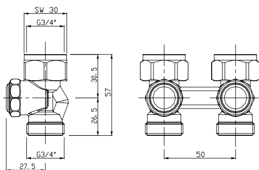
Рис. 2. Прямой для двухтрубных систем.
