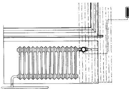
Рис. 4. Установка Thera-2080 с выносным датчиком
