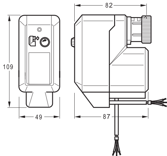
Корпус типа С
